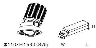
TZ-8736 非調光 L=229・W=53・H=44 TZ-8742K PWM L=267・W=63・H=46
