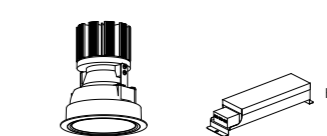
TZ-8728 非調光 L=206・W=51・H=41 TZ-8746K PWM L=228・W=63・H=46 TZ-8758K 位相 L=229・W=53・H=44
