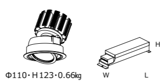
TZ-8736 非調光 L=229・W=53・H=44 TZ-8742K PWM L=267・W=63・H=46
