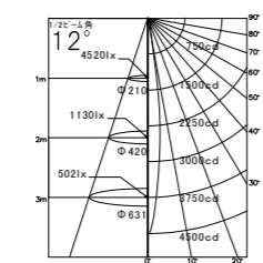
LDR6L-N-E11/D/30/5/12-HC
